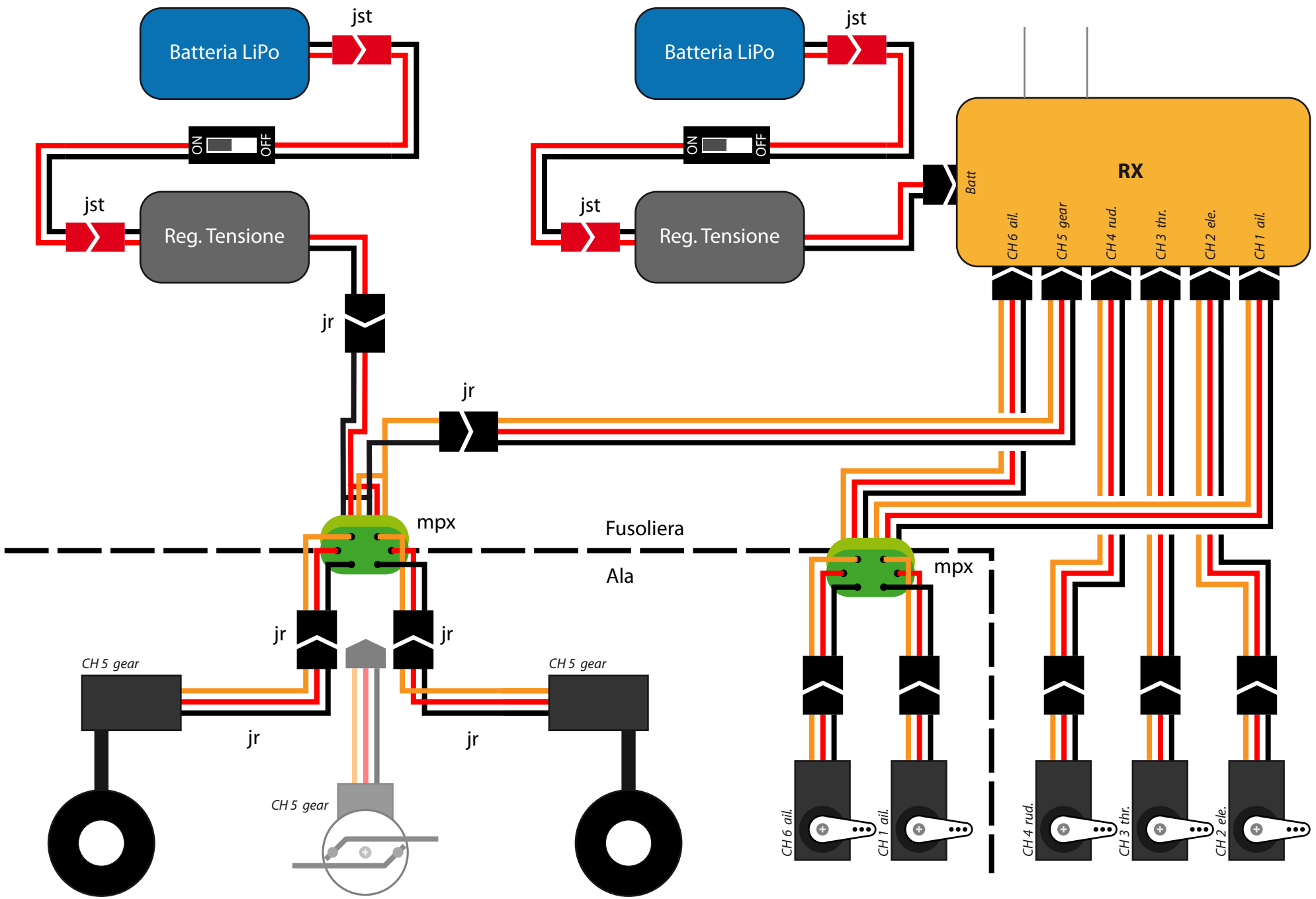
Schema doppia alimentazione e cablaggio servi 2 batterie in fusoliera
