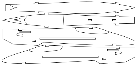
Aile et fuselage dépron 6mm
