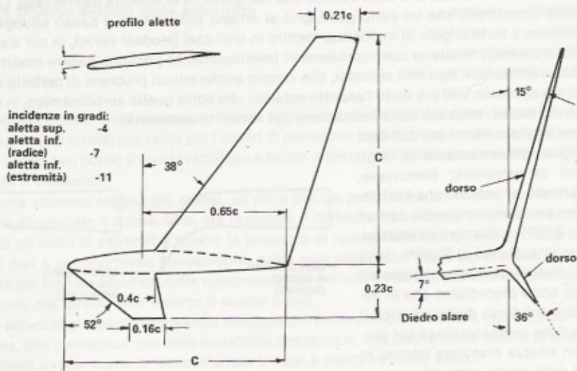
FIG. 6.12 Alette di estremità WHITCOMB (Winglets)
