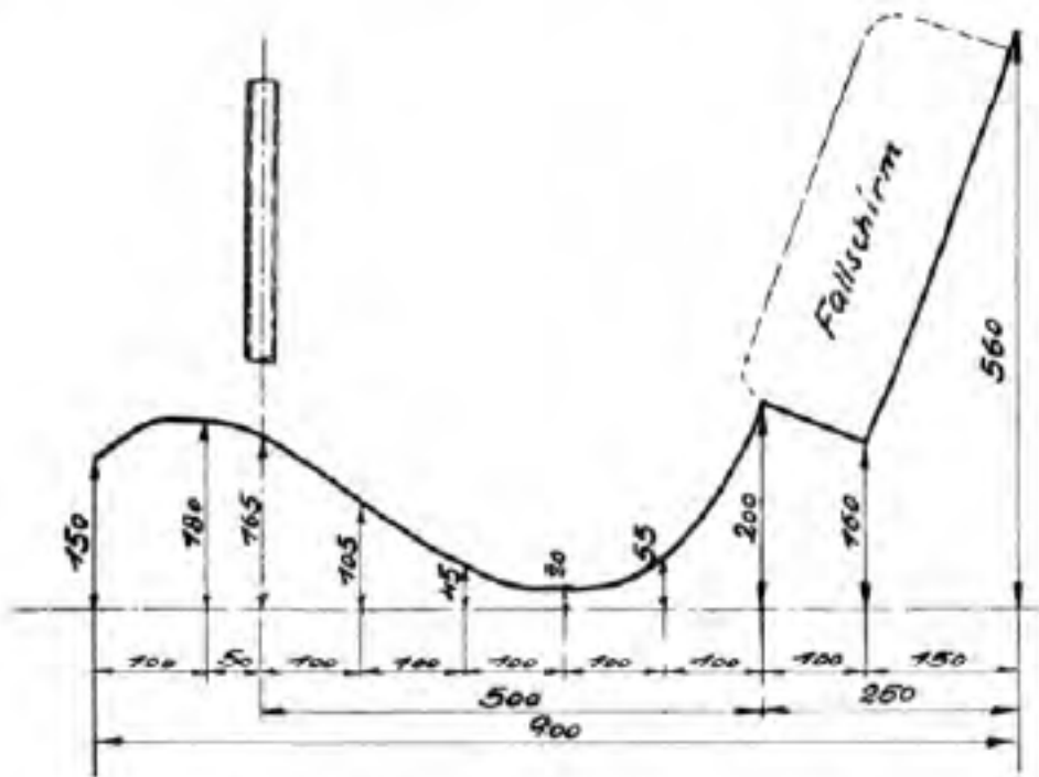
Abb. 124. Maße für einen bequemen Sitz.
